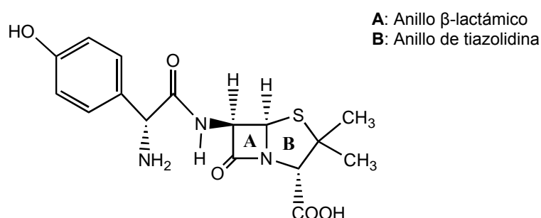
Figura 2. Estructura química de la amoxicilina
